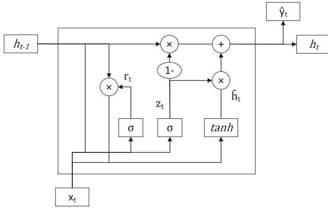
Fig. 6. Default GRU structure.
